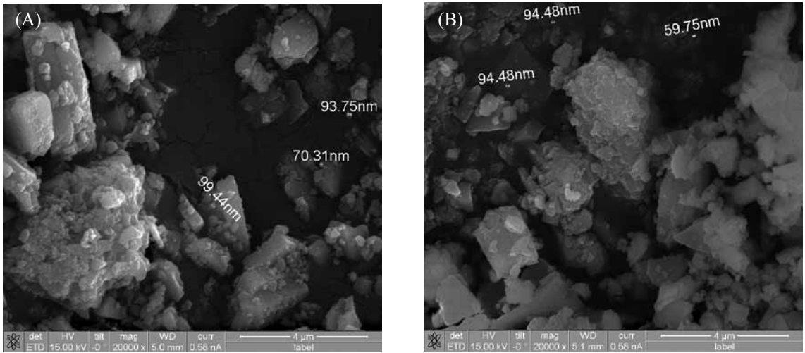
圖四、市售未標示奈米化珍珠粉之掃描式電子顯微鏡 (SEM) 影像。以(A) P1, (B) P2為例
