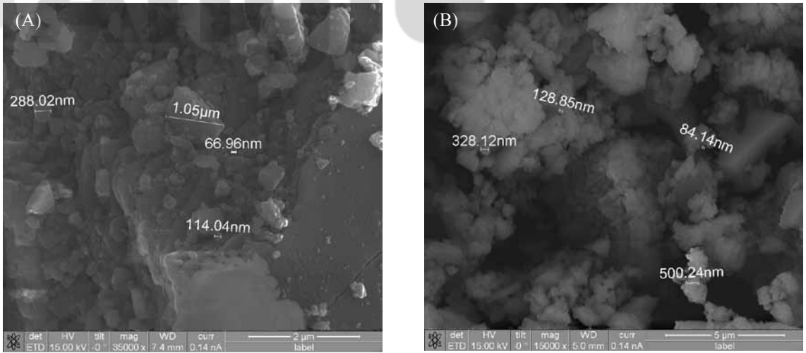
圖三、市售奈米珍珠粉之掃描式電子顯微鏡 (SEM) 影像。以(A) NP1, (B) NP2為例
