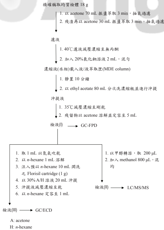
圖一、農產品中農藥多重殘留分析流程
