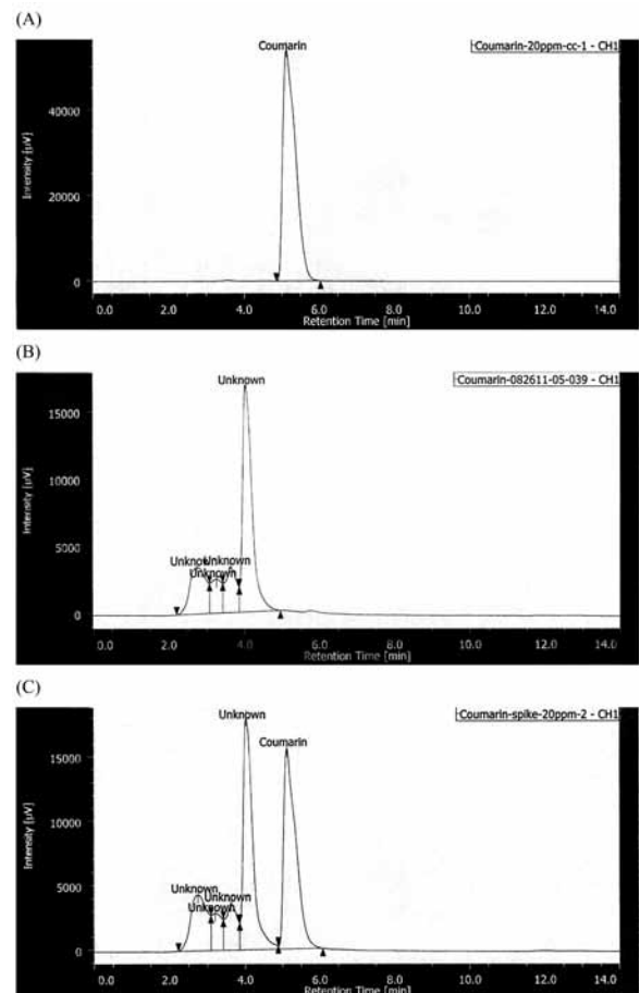
圖二、液相層析圖 (A) 香豆素標準溶液 20 μg/mL、(B) 紅茶檢體及 (C) 紅茶檢體添加香豆素 20 mg/kg
