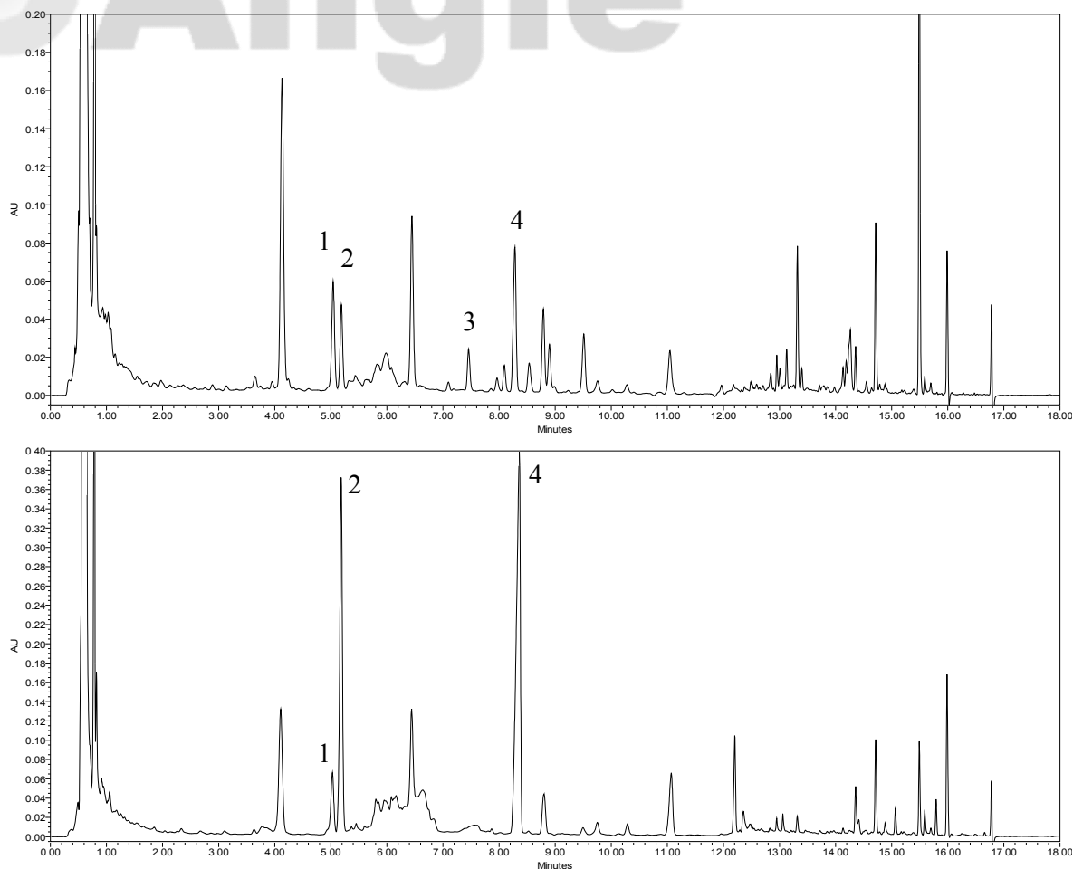
圖七、UPLC 層析圖譜
