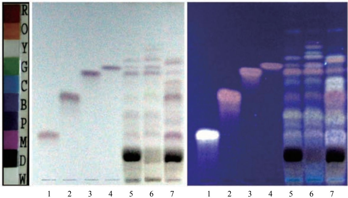
圖六、人參及西洋參藥材薄層層析圖譜
