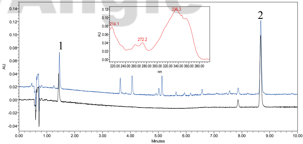
圖五、蒼朮藥材 UPLC 層析圖譜及蒼朮素 UV 圖
