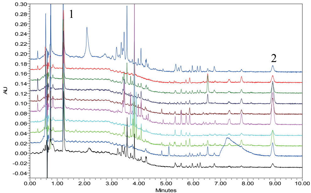
圖六、蒼朮複方濃縮製劑 UPLC 層析圖譜
