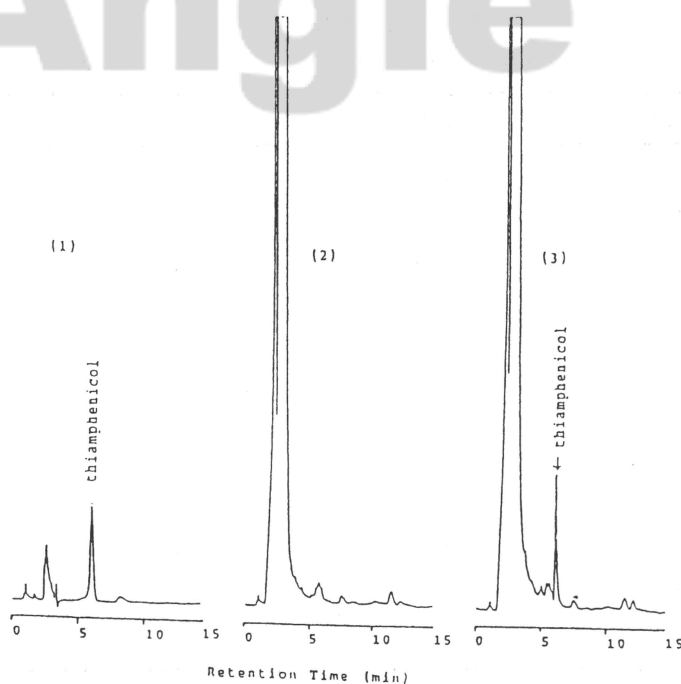
圖三、豬肉中添加甲磺氯黴素回收試驗之液相層析圖
