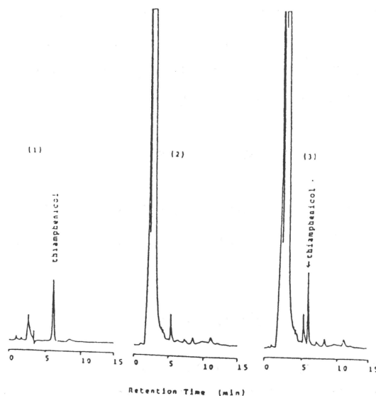
圖四、雞肉中添加甲磺氯黴素回收試驗之液相層析圖
